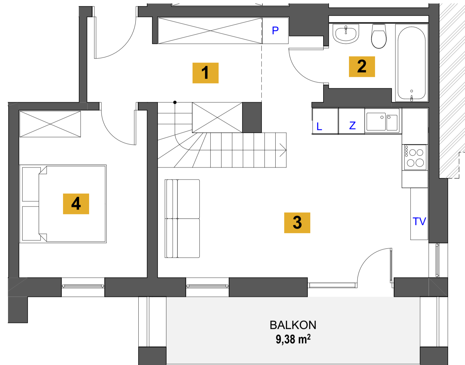
RZUT LOKALU
