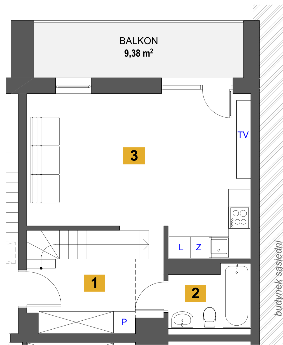
RZUT LOKALU
