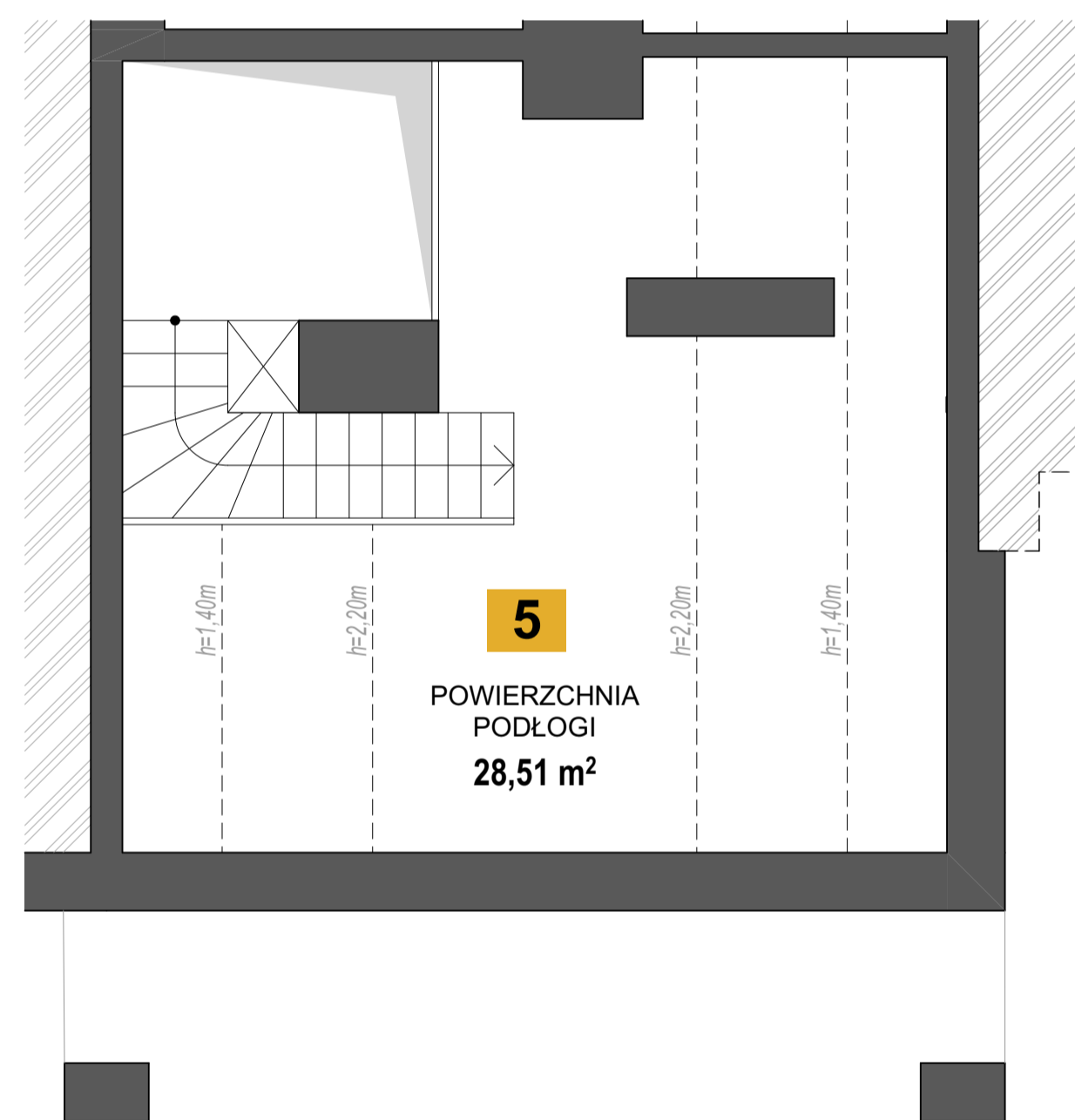
RZUT ANTRESOLI
