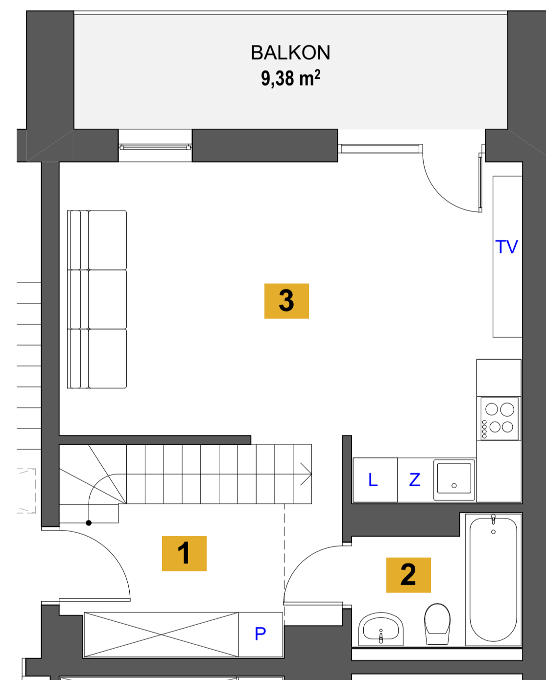
RZUT LOKALU
